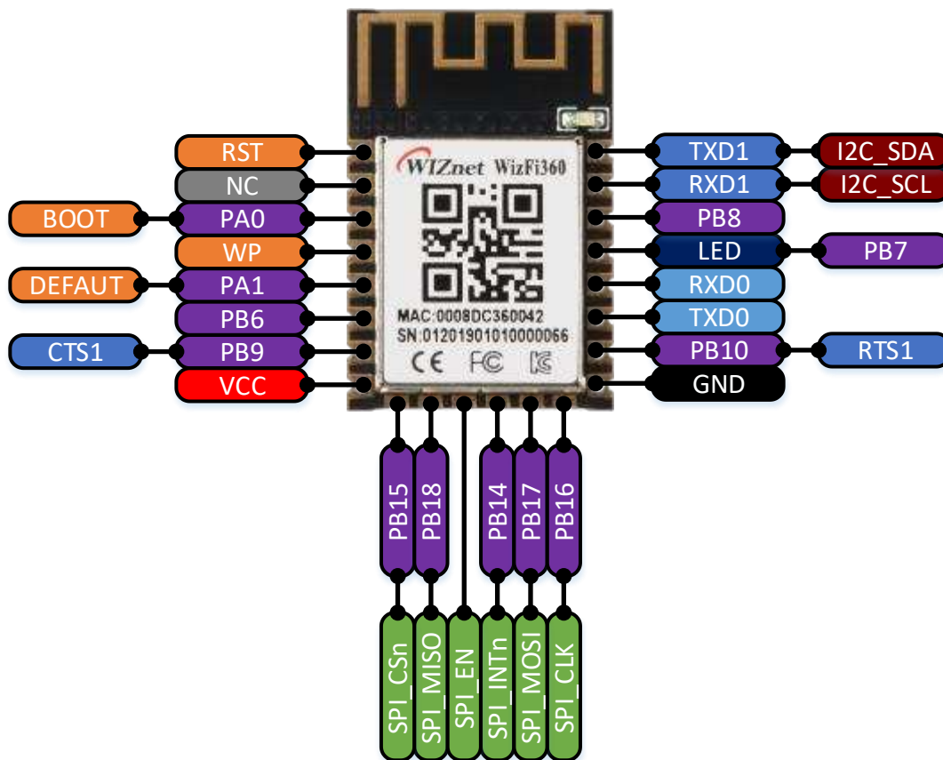
Figure 3. WizFi360 Pinout
