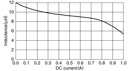
VL4012AT-220MR51
