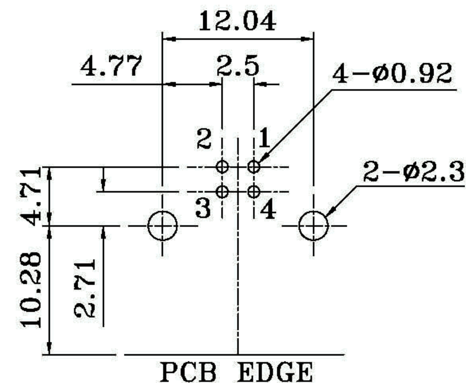
PCB EDGE (COMPONENT SIDE) PCB LAYOUT
