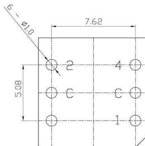
P.C.B DIMENSION
