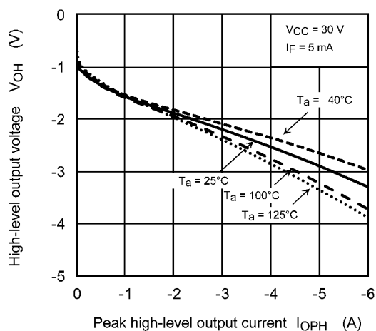
Fig. 12.2.10 V_{OH} - I_{OPH}
