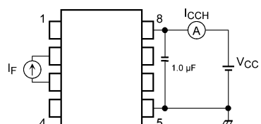
Fig. 12.1.5 I_{CCH} Test Circuit
