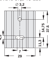
SK 145 37,5 TO 220
