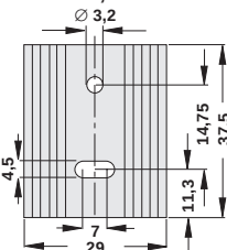
SK 09 37,5 TO 220
