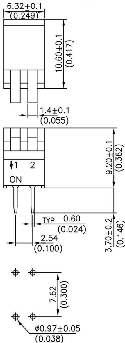
P.C.B. LAYOUT
