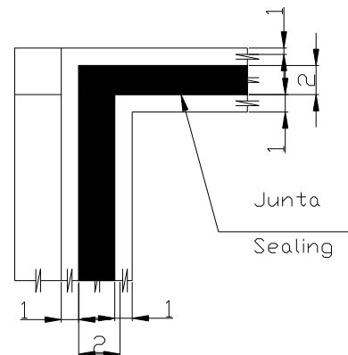
Detalle A
