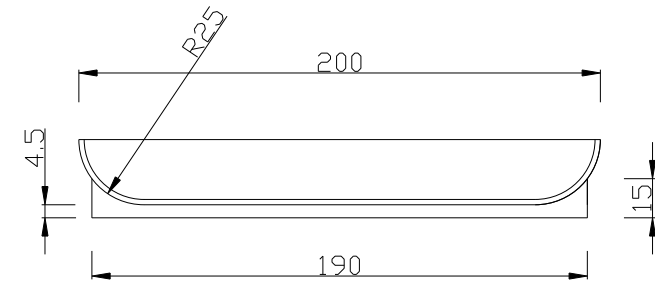
Detalle A
