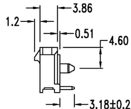
4 ~ 12 circuits
