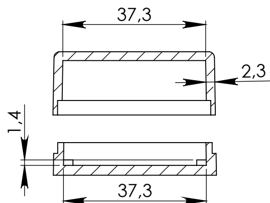
PRZEKRÓJ A-A
