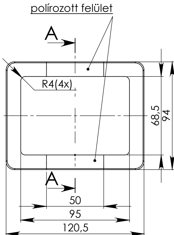
Felülnézet
