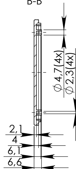
KERESZTMETSZET B-B
