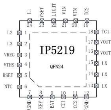
图 2 IP5219 引脚图
