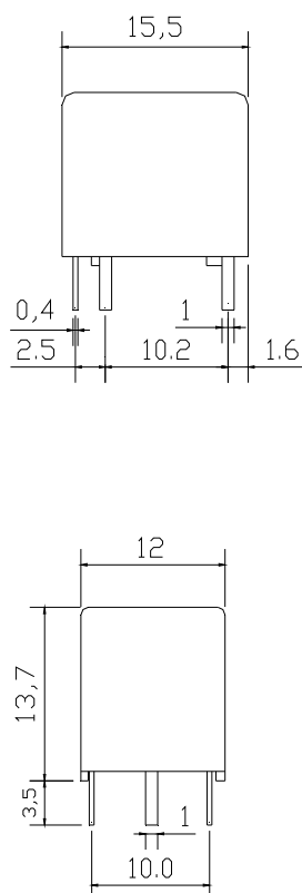
外型图
