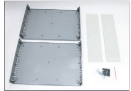
G729V
