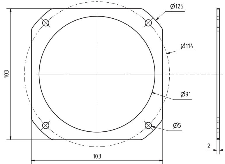
Dichtring/Gasket FRS 10 WP 22.06.2020
