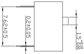
高推钮 (E)
