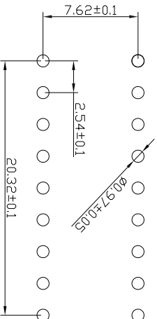
PCB开孔
