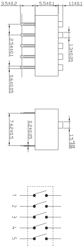
高推钮 (E)
