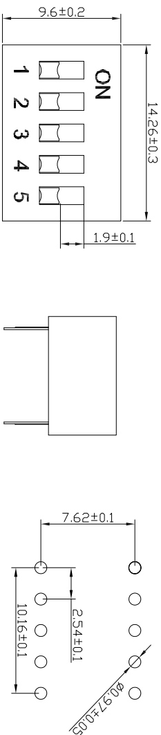
高推钮 (E)
