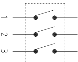
电路图
