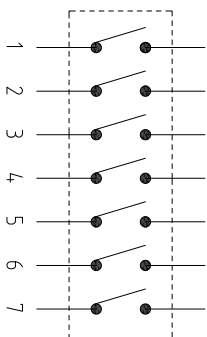
电路图
