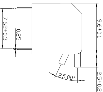
长拨柄 (L)
