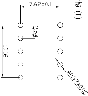
PCB开孔
