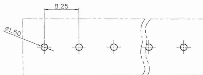
P.C.B LAYOUT
