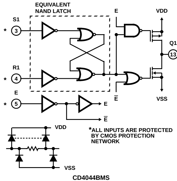
CD4044BMS
