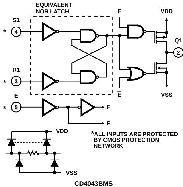
CD4043BMS
