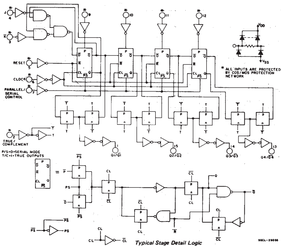
Fig. 4 - Logic diagram.
