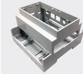
CBRPI-DR
