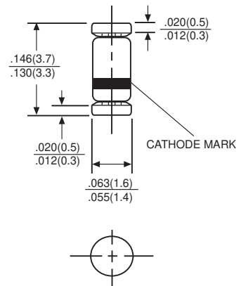
Mini Melf(DL-35)
