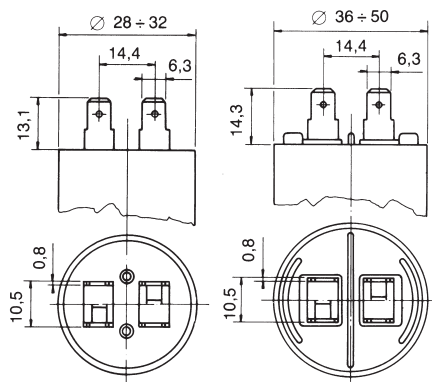
Fig. 1 Doppio Faston 6,35 x 0,8 mm Fig. 1 Double tags 6.35 x 0.8 mm
